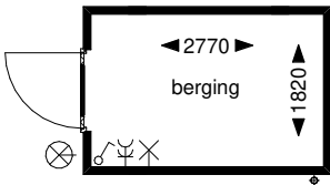
Begane grond
