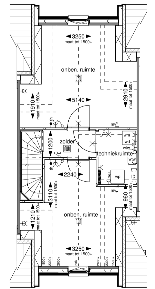
Tweede verdieping
