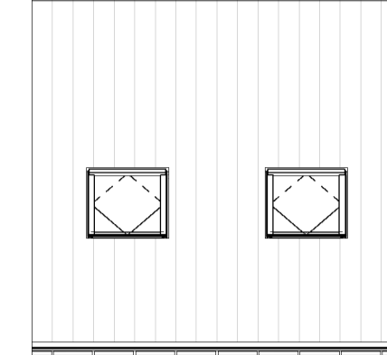
Achtergevel
